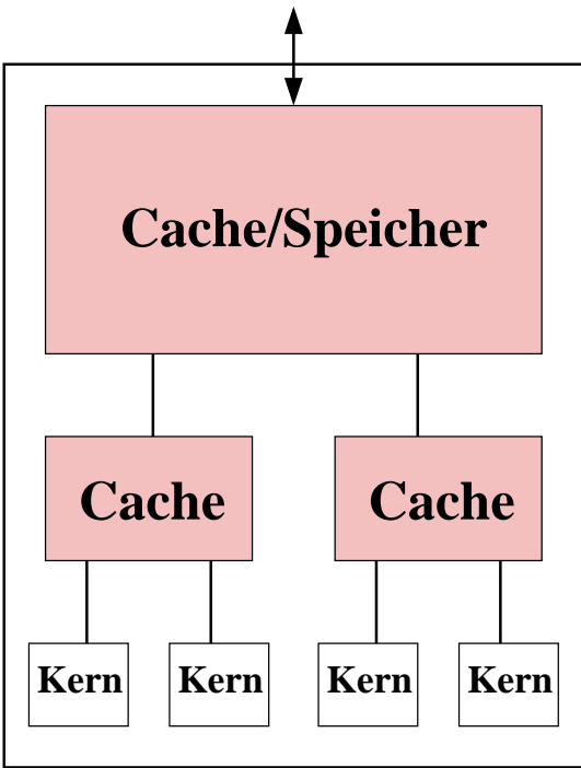
hierarchisches Design
