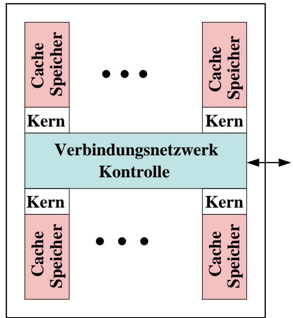
Netzwerkbasierendes Design
