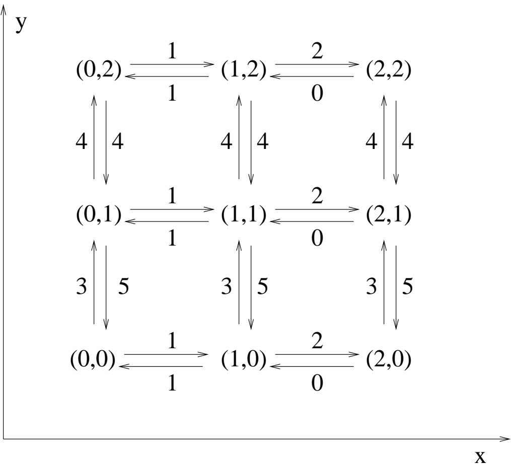
2-dimensionales Gitter mit 3 x 3 Knoten
