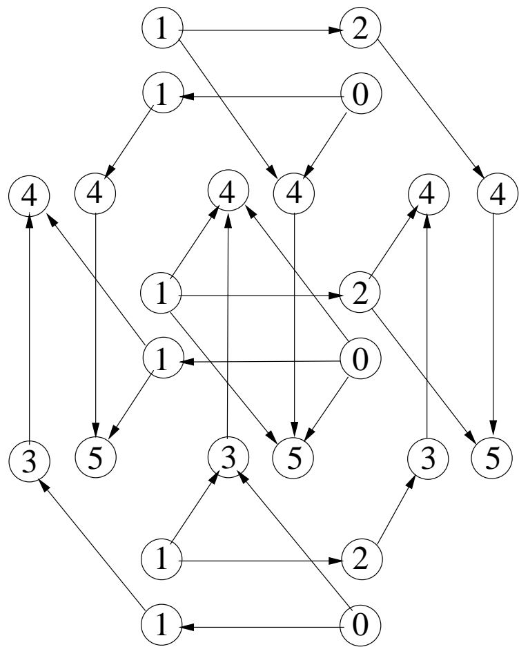
Kanalabhängigkeitsgraph
